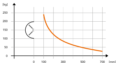
Lastdiagram Axmek VHR 250
